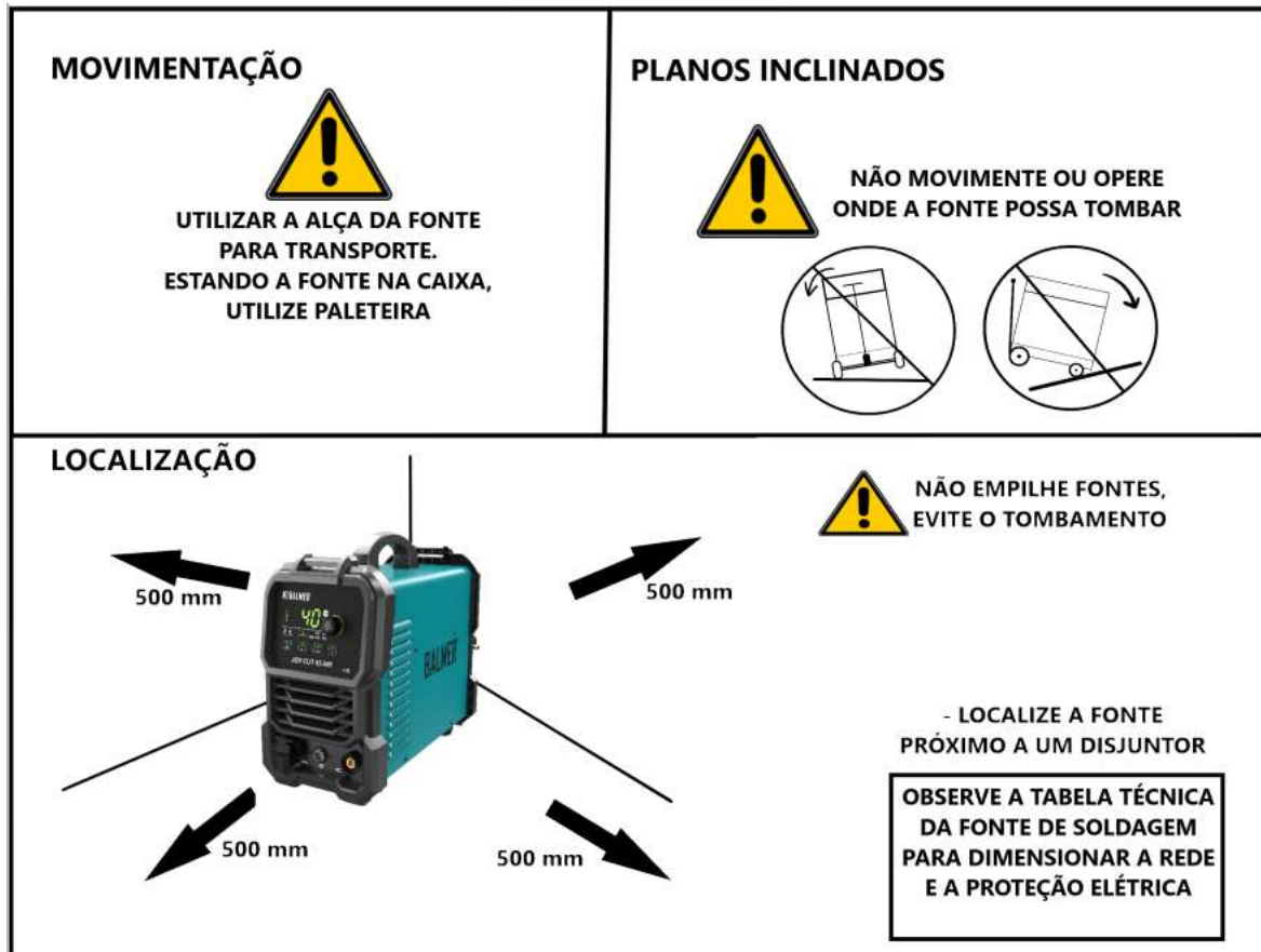
Figura 1 – Atribuição do local de instalação Joy CUT 45 AIR.
